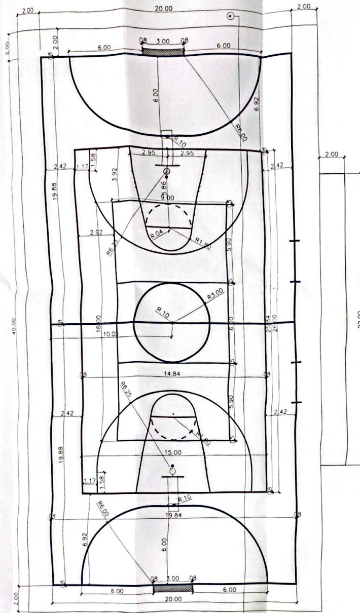
PLANTA ACOTADA ESC.: 1/100
