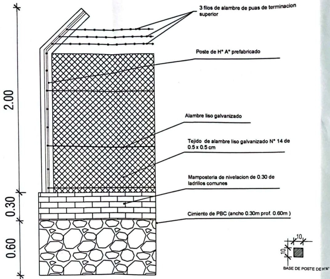
CORTE CERCO PERIMETRAL Esc: 1.20
