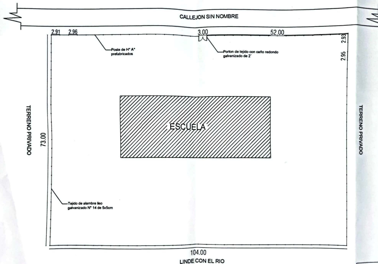
PLANTA DE CERCADO PERIMETRAL Esc: 1/500
