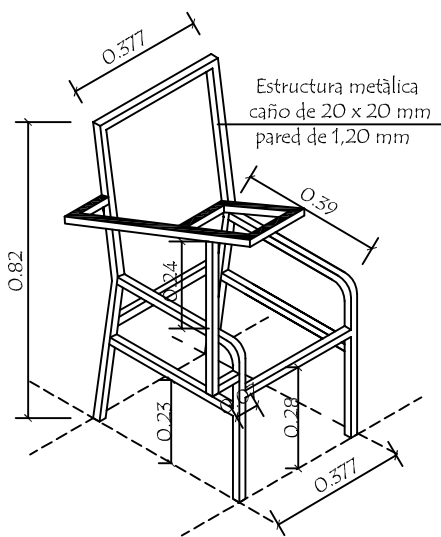
AXONOMETRICA DE ESTRUCTURA METÀLICA
