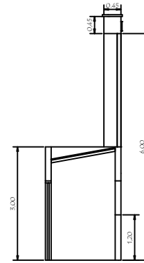
CORTE A
