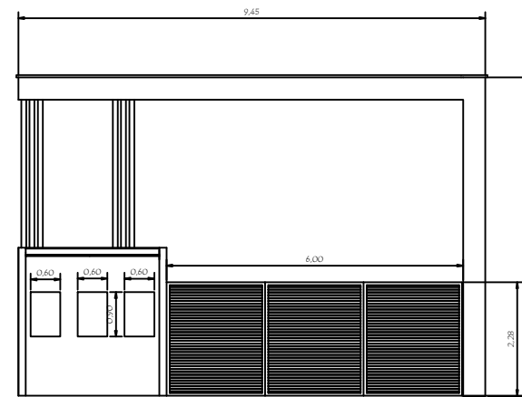
CORTE B
