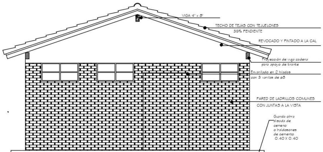
FACHADA
