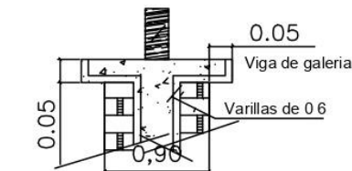
DETALLE CAPITEL
