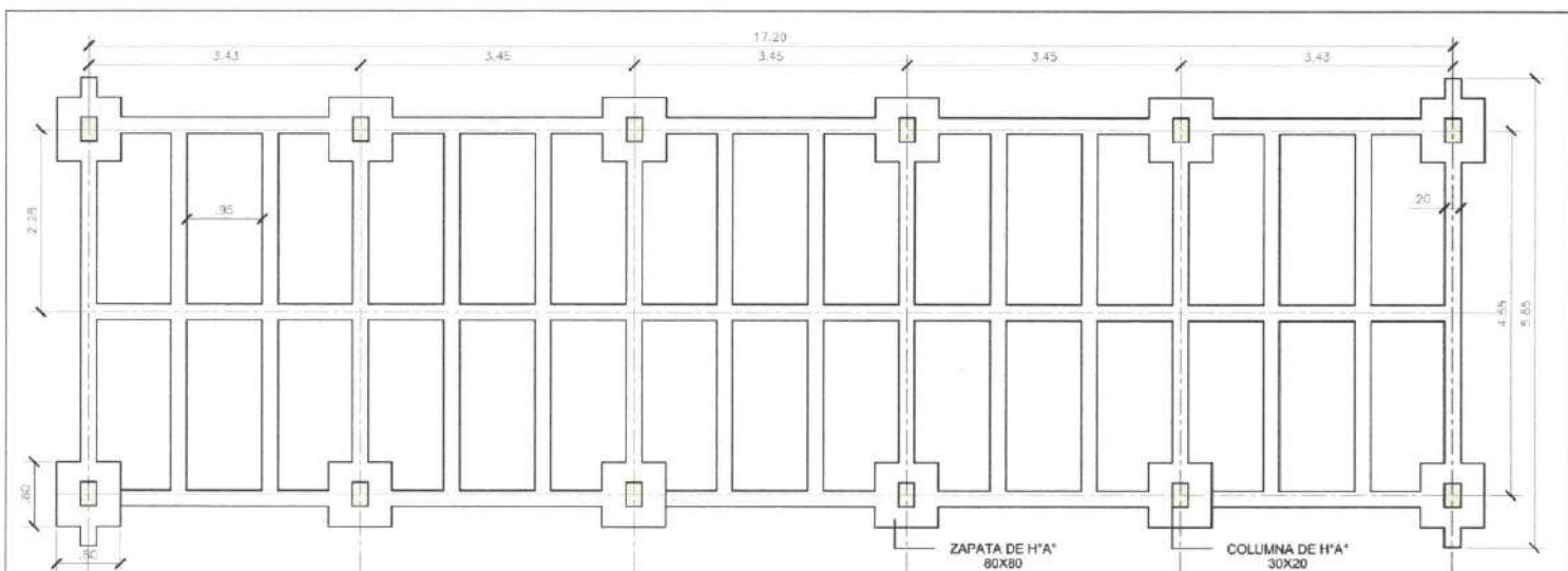
PLANTA DE FUNDACIÓN
