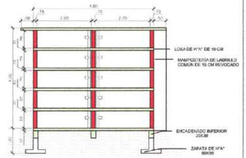
CORTE B-B
