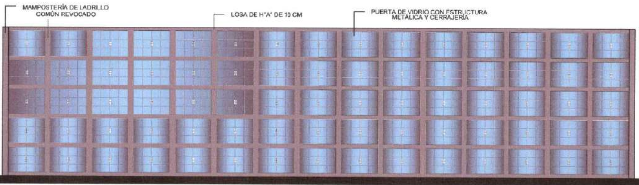
FACHADA FRONTAL
