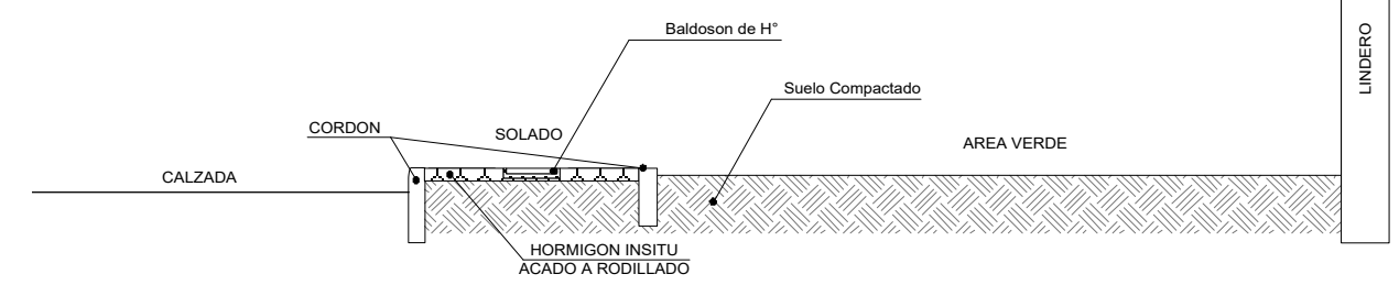
CORTE
