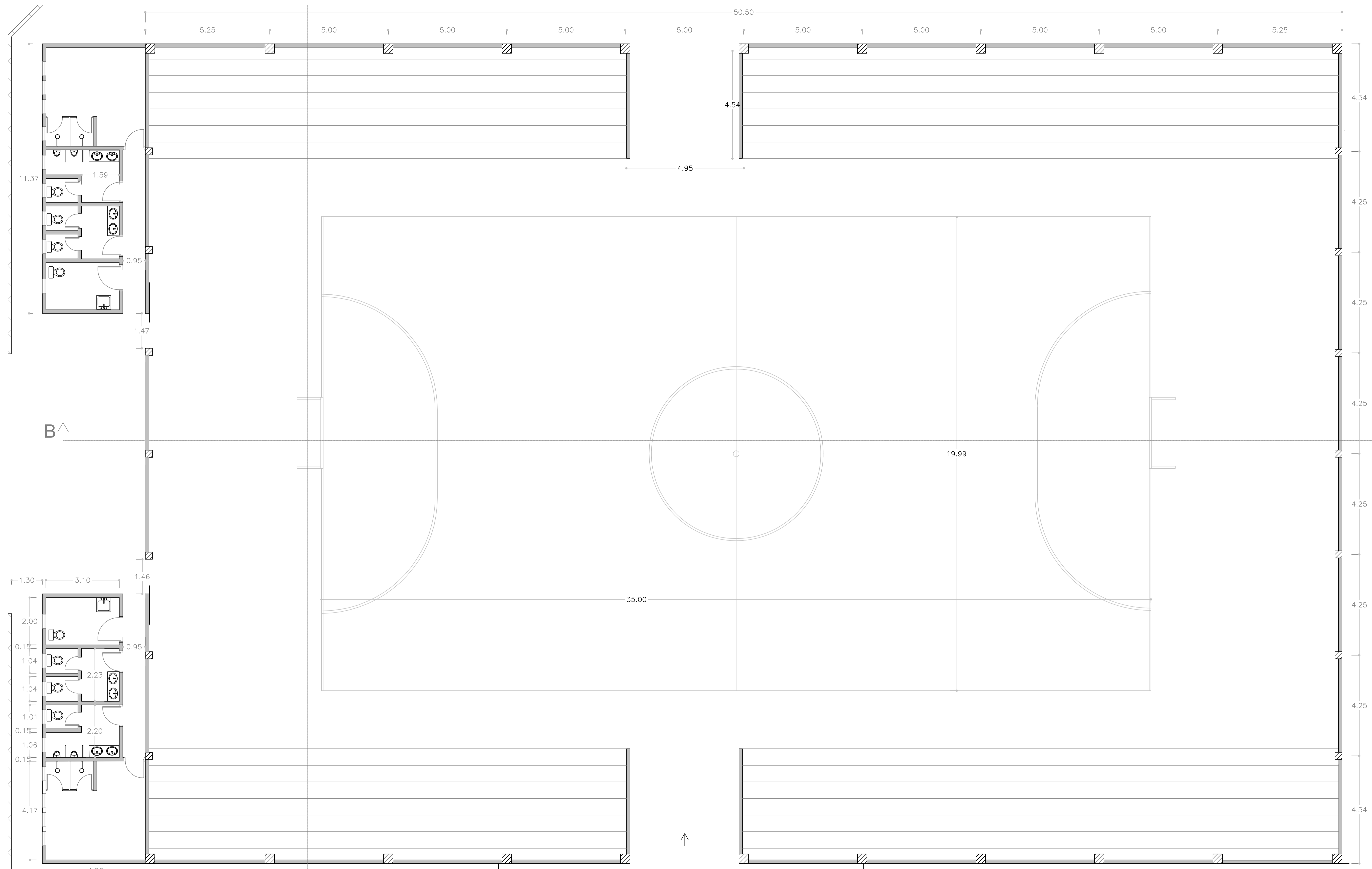
Plano Arquitectonico Acotado Esc. 1/75
